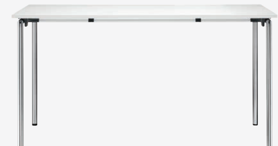
S 1196/2 GESTELL RUNDROHR VERCHROMT, ECKEN AUF GEHRUNG, PLATTE MELAMINHARZBESCHICHTUNG FRAME ROUND TUBE, MITRED CORNERS, CHROME-PLATED, TABLETOP PARTICLE BOARD
